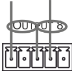
L+ L- G R+ R-
